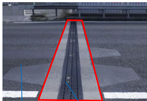
痛んだ継目(伸縮装置)
